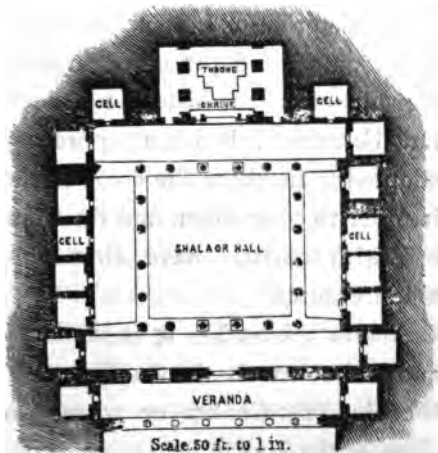
Ajanta Vihâra No. 16.
